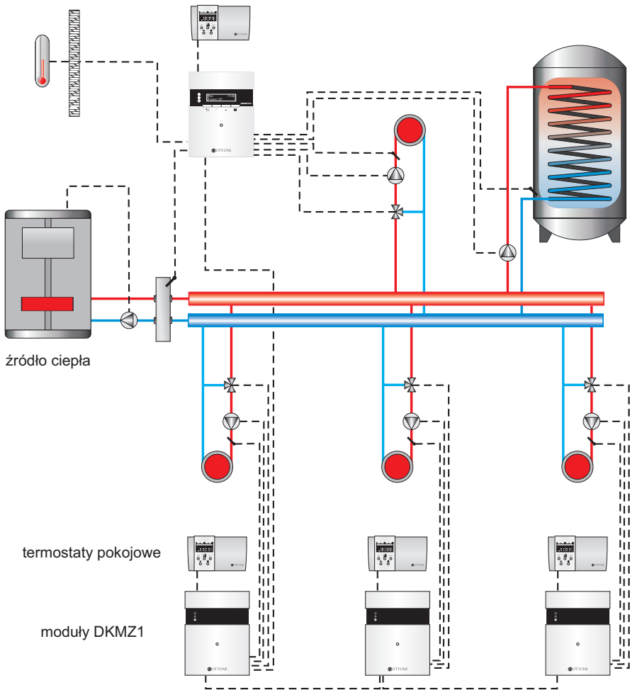
Rys. 2 Przykładowy schemat instalacji z podłączonymi trzema modułami rozszerzającymi DKMZ : Obiegu 3, Obiegu 4 i Obiegu 5. Nie zastępuje on fachowego projektu w miejscu montażu.
