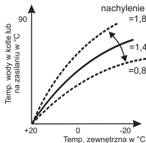
Rys. 12 Nachylenie krzywej grzewczej
