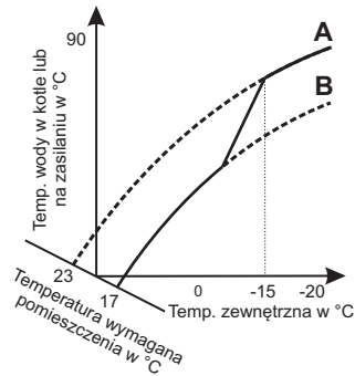
Rys. 11 Zredukowana temp. pomieszczenia
